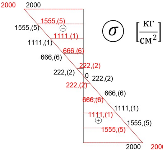
Рис. 4. К примеру 1. Распределение нормальных напряжений \sigma по высоте сечения: черный цвет – аналитический метод; красный цвет – МКЭ
