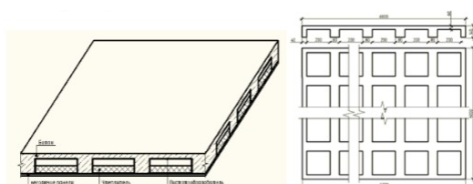
Рисунок 2. - Неизвлекаемые вкладыши-пустотообразователи прямоугольной формы
