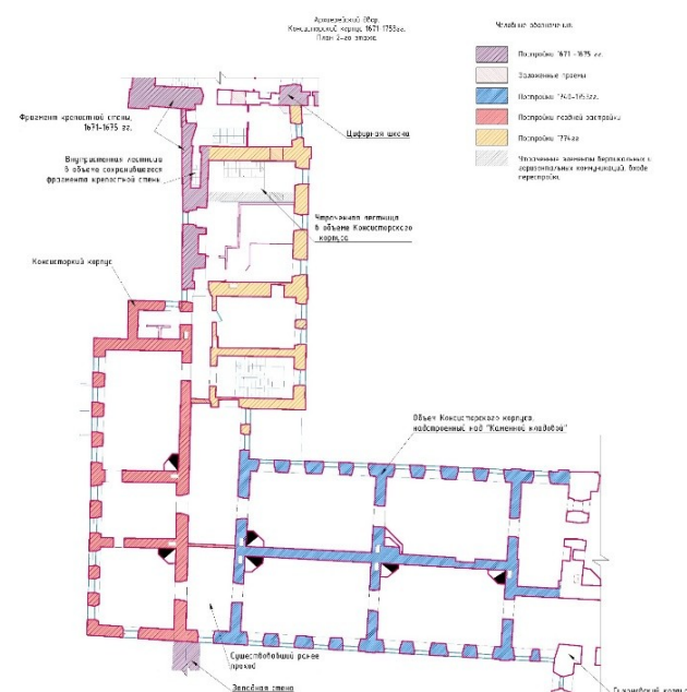
Рисунок 5. Авторская схема строительной периодизации второго яруса.
