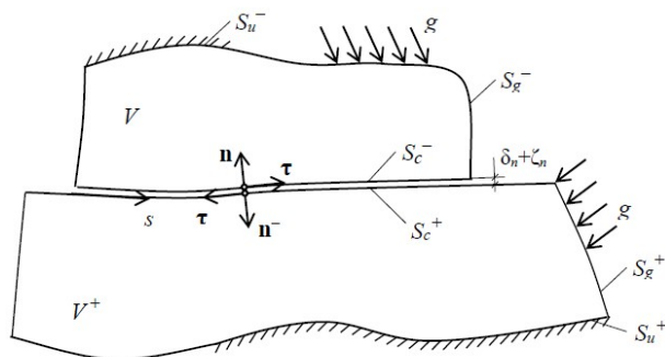
Рисунок 1 - Контактное взаимодействие упруго деформируемых тел
