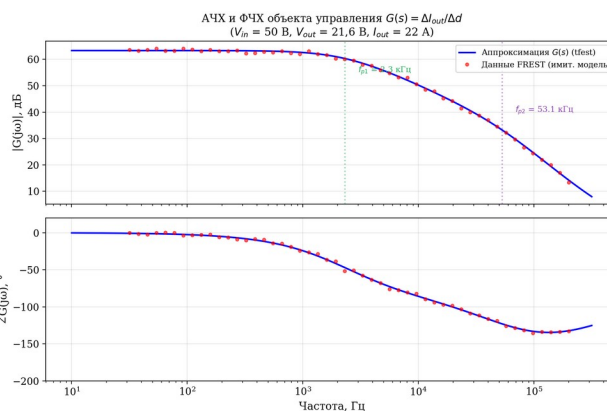
Рисунок 11 — АЧХ и ФЧХ объекта управления G(s) : данные FREST и аппроксимация tfest.
