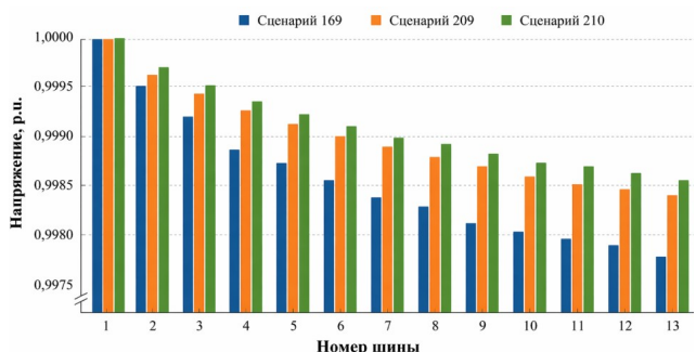
Рисунок 7. Профиль напряжения для лучшего сценария в 13-узловой системе.
