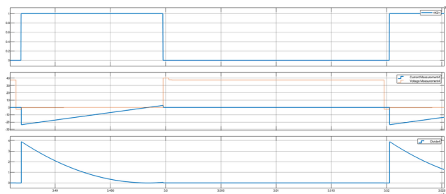
Рисунок 8 — Осциллограммы напряжения управления, VDS, IDS и мощности ключа K2.
