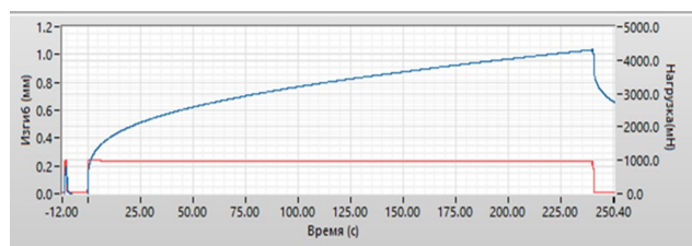
Рисунок 3 – График испытания на реометре BBR.
