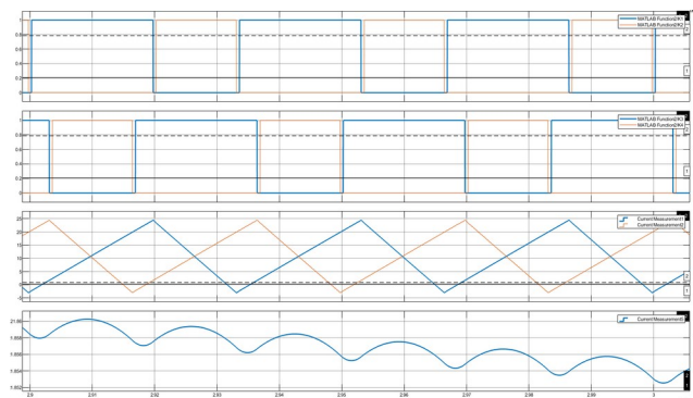
Рисунок 3 — Диаграммы ШИМ-модулятора: опорные пилы, управляющие импульсы, токи фаз и суммарный ток
