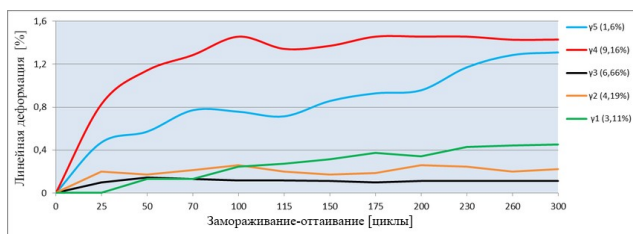
Рис. 2. Линейная деформация бетона после нескольких циклов замораживания-оттаивания [6].
