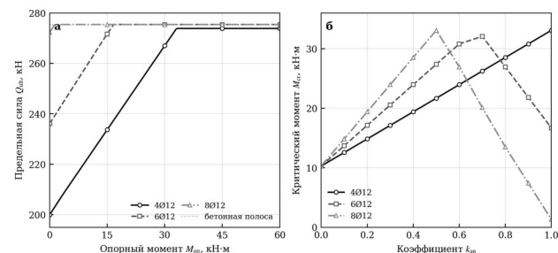
Рис. 2. Результаты расчета: а — зависимость Q_{ult}(M_{on}) при k_{an} = 1 ; б — чувствительность M_{cr} к коэффициенту k_{an}
