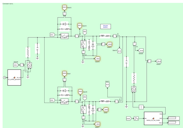
Рисунок 1 — Силовая часть устройства заряда аккумуляторной батареи
