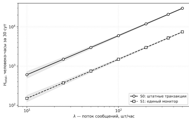
Рисунок 3 – Зависимость суммарной человека-нагрузки от интенсивности потока сообщений \lambda в сценариях S0 и S1
