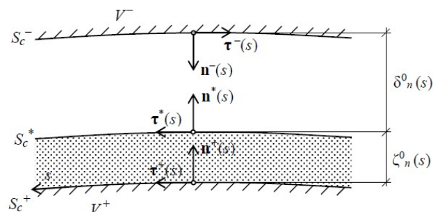
Рисунок 2 - Конфигурация контактного шва
