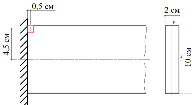
Рис. 1. К определению нормальных напряжений
