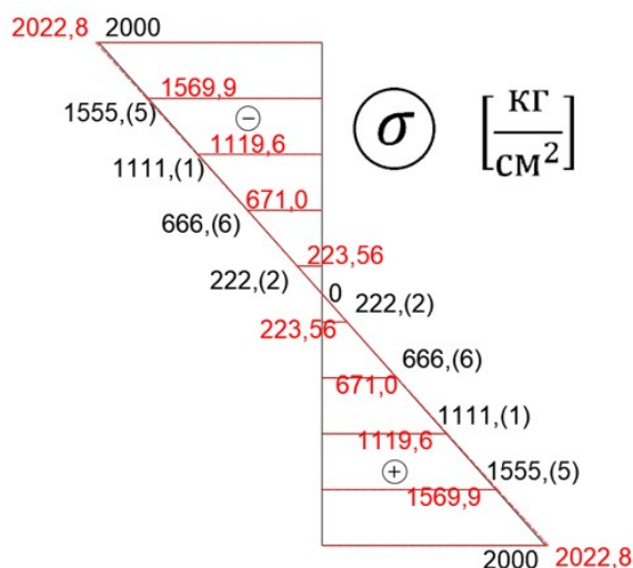
Рис. 10. К примеру 3. Распределение нормальных напряжений \sigma по высоте сечения: черный цвет – аналитический метод; красный цвет – МКЭ
