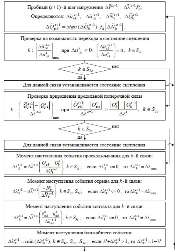
Рисунок 4 – Уточнение методики расчета упругой системы с учетом односторонних связей и трения Кулона
