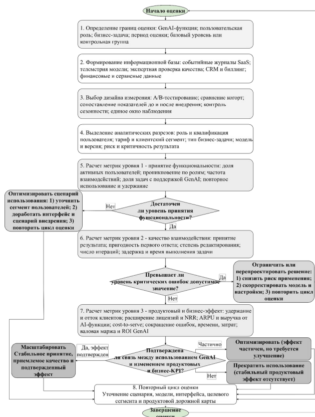
Рисунок 1 – Алгоритм интегрированной оценки эффективности GenAI в B2B SaaS-системах
