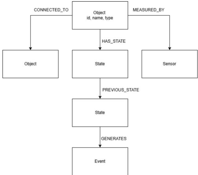
Рисунок 1 – Структура предлагаемой графовой модели данных
