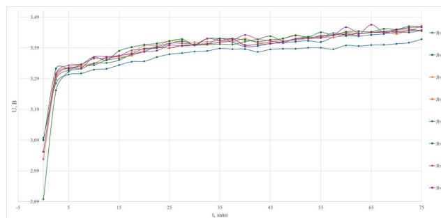
Рис. 7 – Балансировка ячеек аккумуляторной батареи в режиме заряда ( U_{вх} = 29,1 В; I = 2 А)
