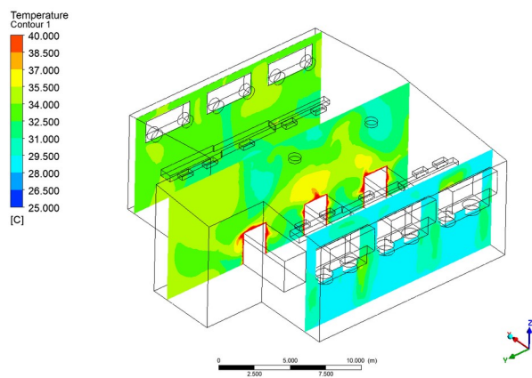
Рисунок 3 - Поле распределения температур. Продольные сечения
