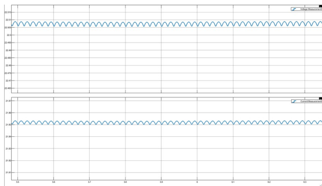
Рисунок 4 — Выходной ток и напряжение в установившемся режиме CC
