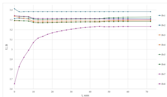
Рис. 5 – Балансировка ячеек аккумуляторной батареи при одной существенно разряженной ячейке
