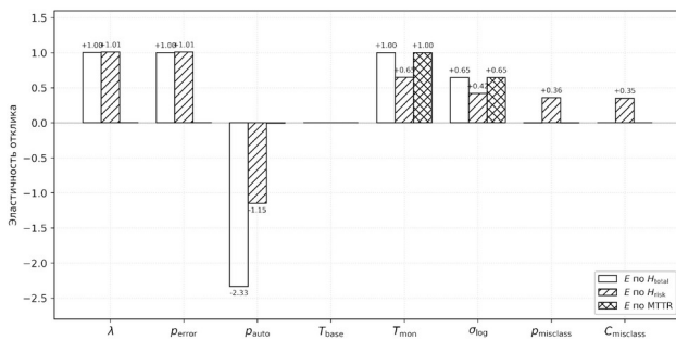
Рисунок 4 – Частные эластичности целевых метрик H_{total} , H_{risk} и MTTR по параметрам модели в окрестности рабочей точки
