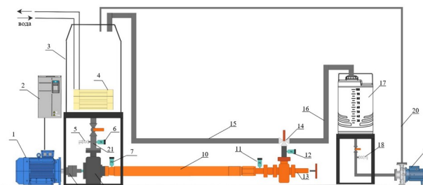
Рисунок 1. Принципиальная схема испытательного стенда.
