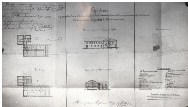
Рисунок 3. Копия чертежа. «Проект переустройства и предполагаемой каменной пристройки для лестницы Вологодской Духовной Консистории», 1893 г. ГАВО, ф. 1293, оп. 126, д. 69.
