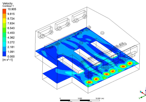
Рисунок 2 - Поле распределения скоростей. Высота – 2 м
