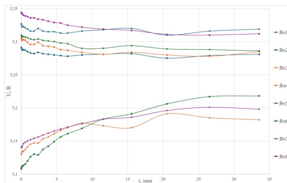
Рис. 4 – Балансировка ячеек аккумуляторной батареи при исходном разбросе напряжений
