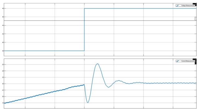
Рисунок 14 — Переходный процесс при повышении входного напряжения с 38 В до 48 В
