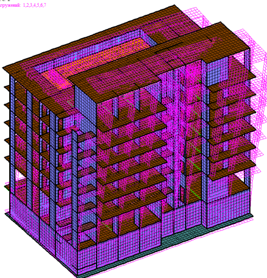
Рисунок 7. - колебания при 2 периоде
