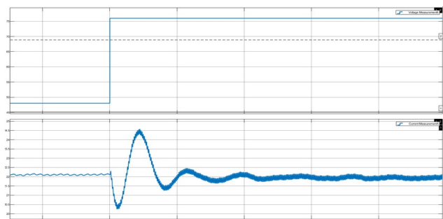
Рисунок 15 — Переходный процесс при повышении входного напряжения с 48 В до 76 В
