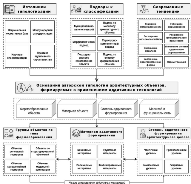
Рисунок 1 – Авторская схема типологии архитектурных объектов, формируемых с применением аддитивных технологий
