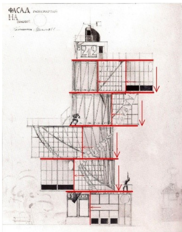
Рис.2. Проект Московского отделения газеты Ленинградская правда, 1924 г. Схема стыковки конструктивных сеток (а) проект К.С. Мельникова)
