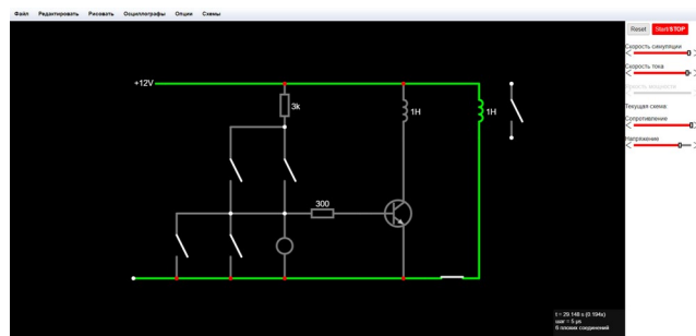
Рис. 9 – Схема в программе FALSTAD
