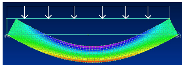
Рис. 9. К примеру 3. Расчетная схема. Пластиночная модель
