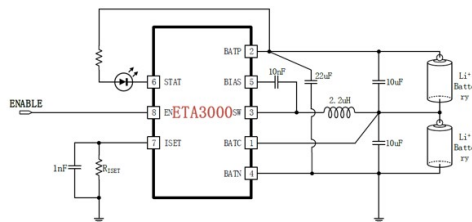
Рис. 1 – Схема подключения микросхемы ЕТА3000 к двум соседним аккумуляторным ячейкам
