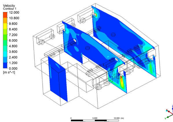
Рисунок 6 - Поле распределения скоростей. Поперечные сечения
