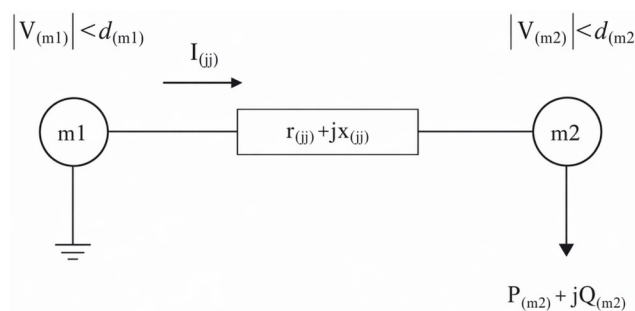
Рисунок 2. Типовая радиальная сеть.
