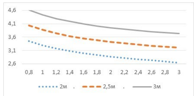
Рис. 4. Отношение площадей при 45^\circ
