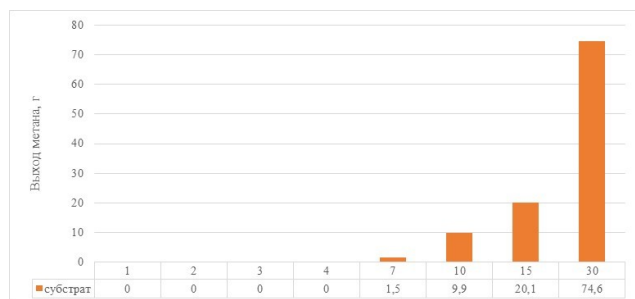
Рисунок 8 – Потенциал метанообразования
