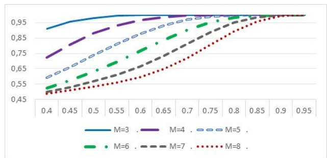
Рис. 9. Вероятность не менее M успехов подряд в 20 испытаниях
