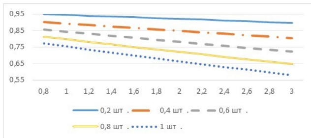
Рис. 7. Вероятность P_0(0) для вездехода длины 2 м
