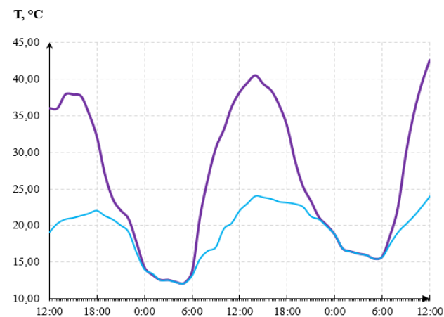
Рис.2 Осциллограммы суточного изменения температуры за период 26.06.2025-28.06.2025
