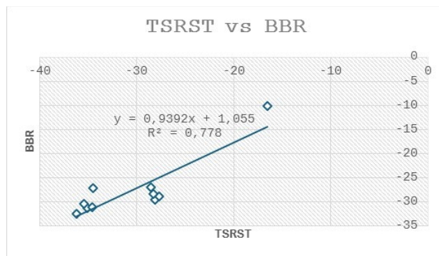
Рисунок 2. Зависимость критической температуры по параметру m (BBR) от температуры трещинообразования по TSRST
