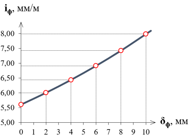
Рис. 4 График зависимости i_{\phi}=f(\delta_{\phi})
