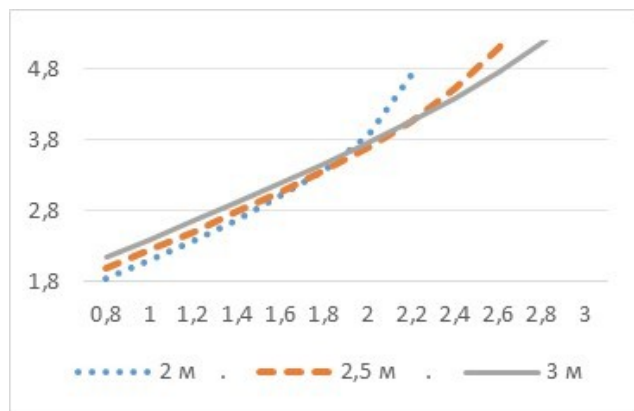
Рис. 2. Средняя необходимая площадь при 60^\circ
