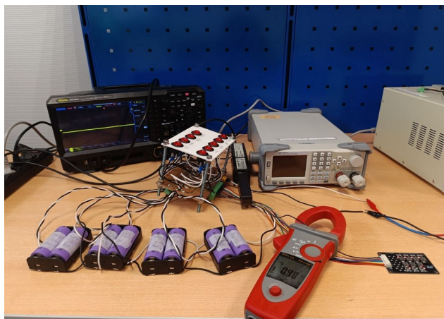
Рис. 3 – Внешний вид экспериментального макета контроллера активной индуктивной балансировки аккумуляторной батареи
