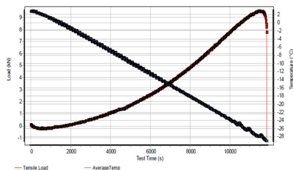
Рисунок 2 – График изменения температуры и растягивающего усилия в процессе испытания образца
