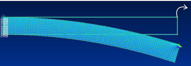
Рис. 6. К примеру 2. Расчетная схема. Пластиначая модель
