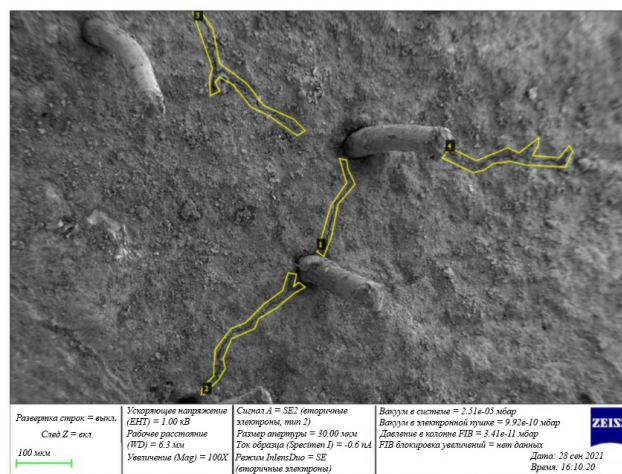
Рис. 3. Аннотированное изображение 1, 2, 3, 4 — порядковые номера трещин (присвоены автоматически при разметке) [8].
