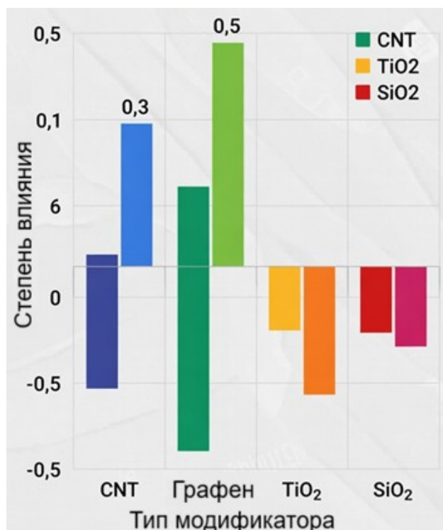
Рис. 5. – Гистограмма степени влияния модификаторов на механические свойства полиэтиленовых труб (коэффициенты регрессии b i , нормированные)
