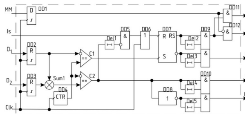
Рисунок 4 – Функциональная схема цифрового модулятора
