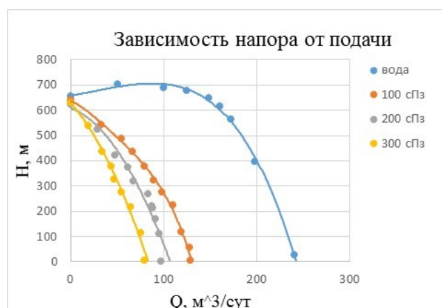
Рисунок 2. Зависимость напора от подачи для насоса ЭЦН5А-160 при работе на воде и средах с вязкостью 100, 200, 300 сПз
