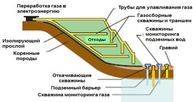
Рисунок 1. Современные технологии мониторинга и защиты грунтовых вод.
