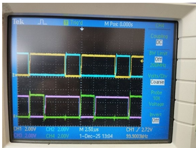
Рисунок 6 – Осциллограмма выходных импульсов модулятора
