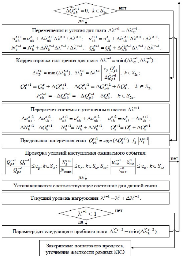
Рисунок 4, продолжение – Уточнение методики расчета упругой системы с учетом односторонних связей и трения Кулона
