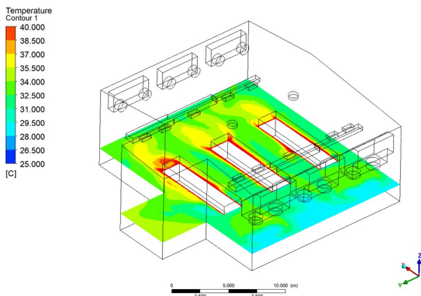
Рисунок 1 - Поле распределения температур. Высота – 2 м
