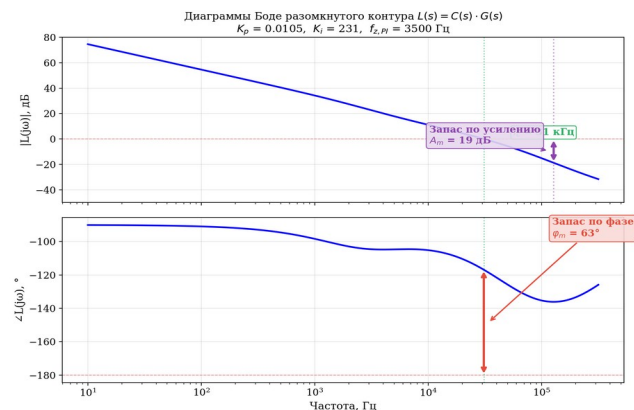
Рисунок 12 — Диаграммы Бode разомкнутого контура L(s) = C(s) \cdot G(s)
