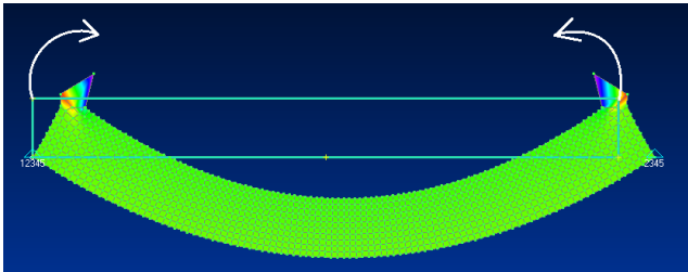
Рис. 3. К примеру 1. Расчетная схема. Пластиначая модель
