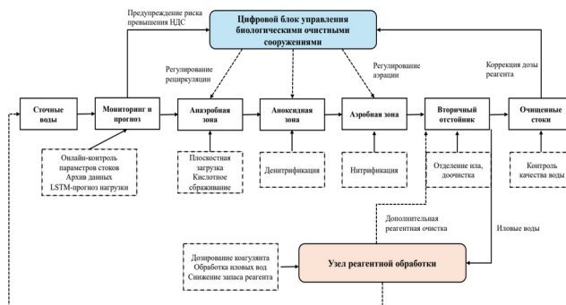
Рисунок 1. Структура модели модернизации аэротенка для снижения капитальных и эксплуатационных затрат ОВКХ при соблюдении НДС по соединениям азота и фосфора
