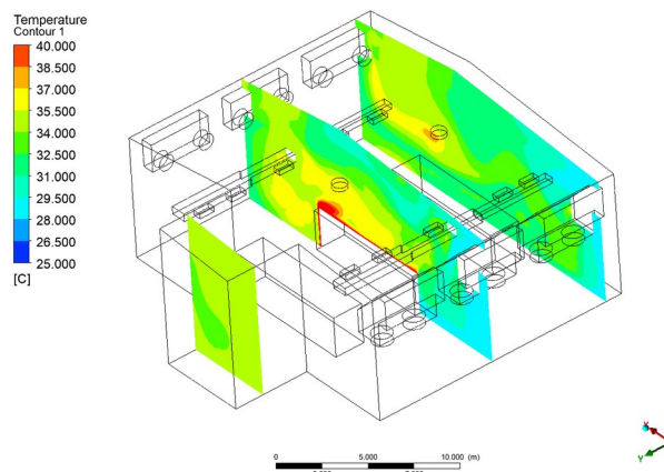
Рисунок 4 - Поле распределения температур. Поперечные сечения
