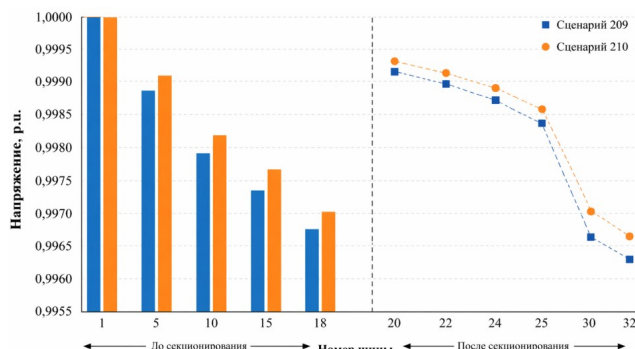
Рисунок 5. Сравнение профилей напряжения для сценариев 209 и 210.
