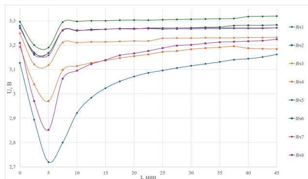
Рис. 6 – Балансировка ячеек аккумуляторной батареи в режиме разряда
