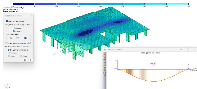
Рисунок 5. – Прогиб монолитной плиты перекрытия
