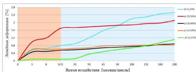
Рис. 1. Деформация бетонов, подвергнутых воздействию раствора \text{Na}_2\text{SO}_4 и последующим циклам замораживания-оттаивания [6].
