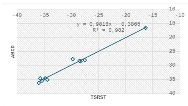
Рисунок 1. Зависимость температуры растрескивания по ABCD от температуры трещинообразования по TSRST
