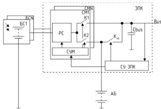
Рисунок 1 – Структурная схема энергопреобразующего комплекса
