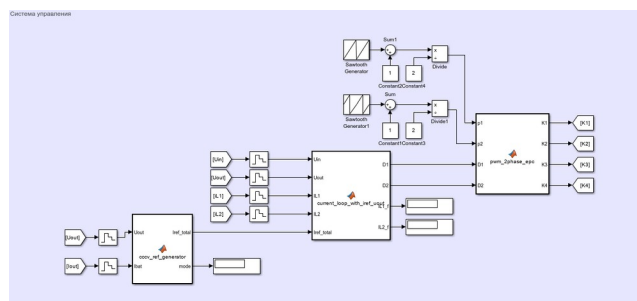
Рисунок 2 — Система управления устройством заряда аккумуляторной батареи
