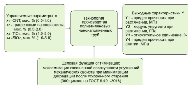
Рис. 4. – Параметры состава и структуры полиэтиленовых труб с нанодобавками для оперативной оценки их механических свойств
