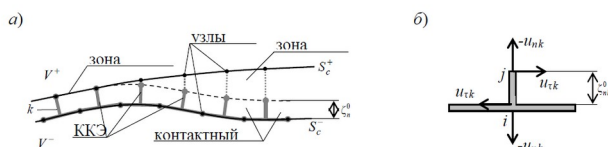
Рисунок 3 - Схема контактного взаимодействия при односторонних связях с трением Кулона
