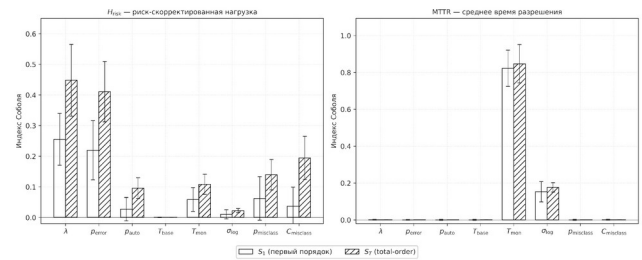
Рисунок 5 – Индексы Соболя первого порядка S_1 и total-order S^T для целевых метрик H_{risk} и MTTR
