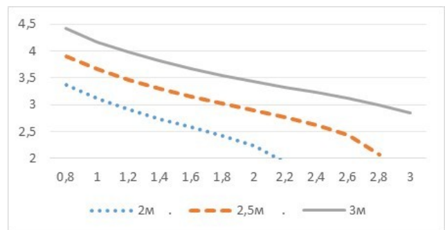
Рис. 5. Отношение площадей при 60^\circ
