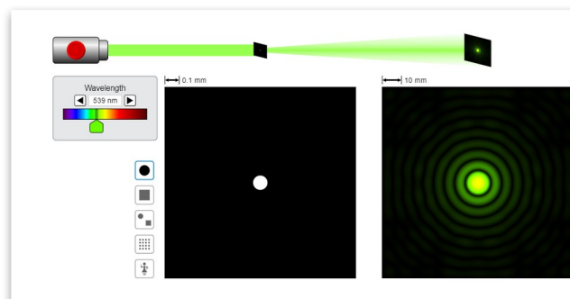
Рис. 8. Определение по дифракции
