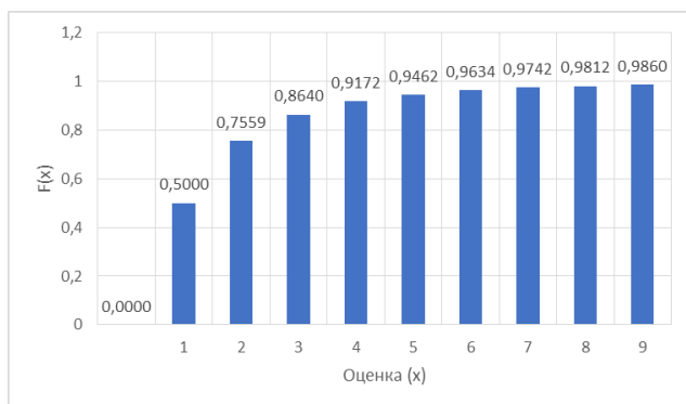
Рис. 1. Гистограмма функции распределения логнормального закона.
