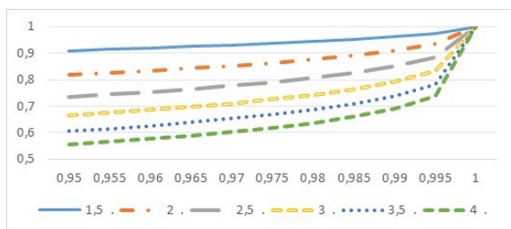
Рис. 11, а. Необходимая вероятность шага при малом выборе
