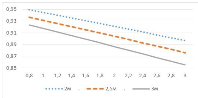
Рис. 6. Шансы, что единственный участок свободен при плотности 0,2
