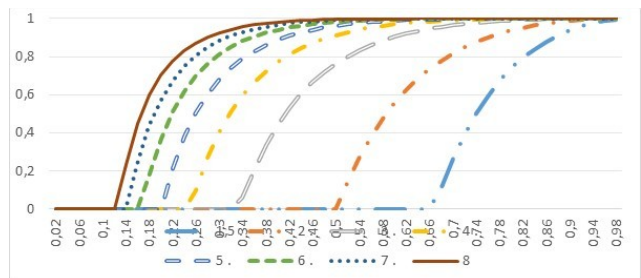
Рис. 10. Проходимость P_* в зависимости от P_l и от r = S_{дост} / S_{ср}
