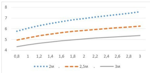
Рис. 8. Необходимое число свободных участков
