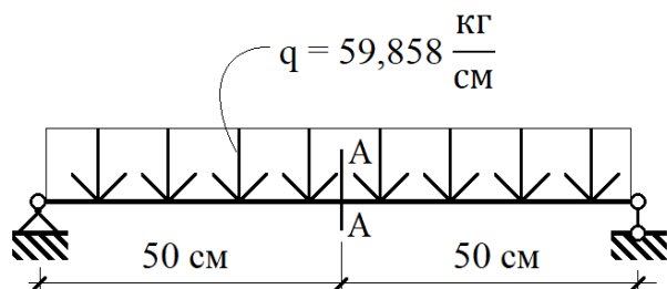
Рис. 8. К примеру 3. Расчетная схема
