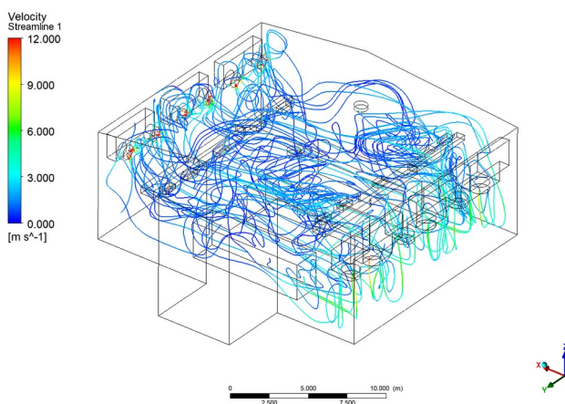
Рисунок 7 - Линии тока
