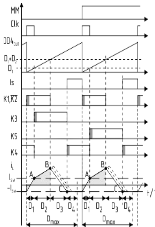
Рисунок 5 – Диаграммы работы модулятора и тока дросселя ЧППП
