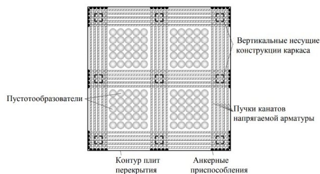
Рисунок 1. - Схема облегченного постнапряженного перекрытия.
