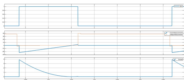
Рисунок 10 — Осциллограммы напряжения управления, VDS, IDS и мощности ключа K4
