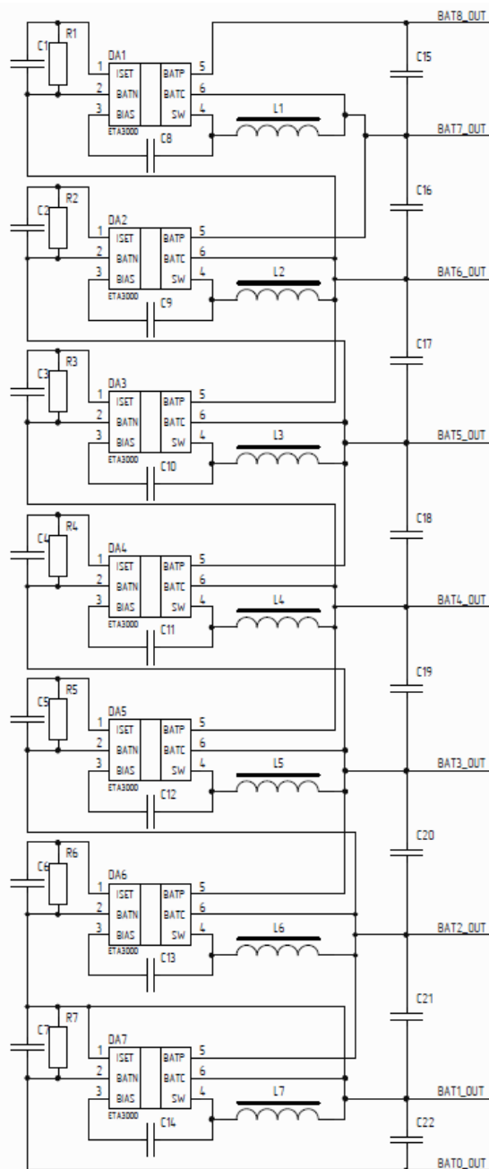
Рисунок 2 - Подключение микросхем ETA3000 для восьмизлементной аккумуляторной батареи
