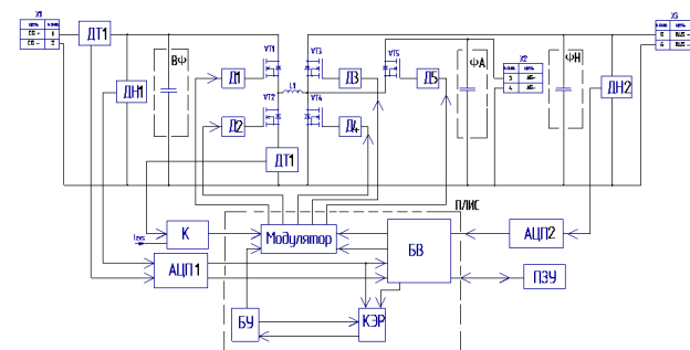
Рисунок 3 – Функциональная схема ЭПК
