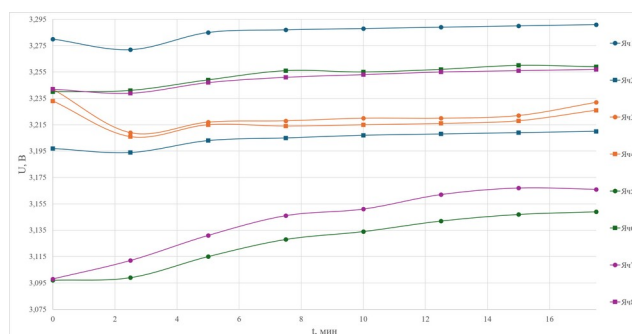
Рис. 8. Балансировка ячеек аккумуляторной батареи в буферном режиме ( I_{бал} \approx 0,25 А)
