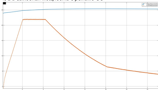
Рисунок 6 — Переход из режима CC в режим CV: выходное напряжение и ток
