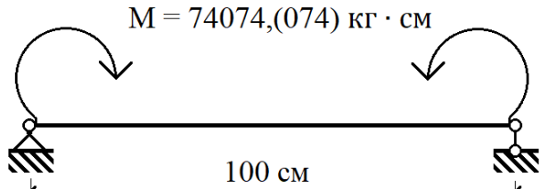
Рис. 2. К примеру 1. Расчетная схема
