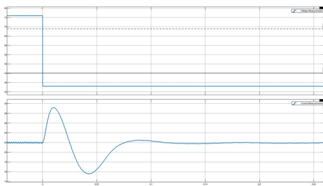
Рисунок 16 — Переходный процесс при понижении входного напряжения с 76 В до 38 В
