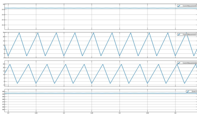
Рисунок 5 — Суммарный выходной ток, токи дросселей фаз 1, 2 и выходная мощность в режиме CC
