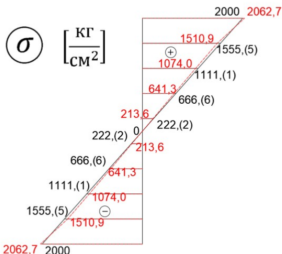
Рис. 7. К примеру 2. Распределение нормальных напряжений \sigma по высоте сечения: черный цвет – аналитический метод; красный цвет – МКЭ
