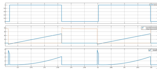
Рисунок 7 — Осциллограммы напряжения управления, VDS, IDS и мощности ключа K1.
