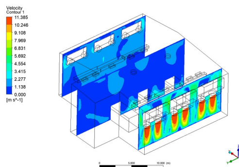
Рисунок 5 - Поле распределения скоростей. Продольные сечения
