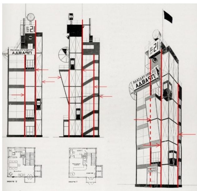
Рис.3. Проект Московского отделения газеты Ленинградская правда, 1924 г. Схема стыковки конструктивных сеток. (б) проект В.А. и А.А. Весниных))
