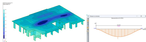
Рисунок 9. – Прогиб пустотной плиты перекрытия
