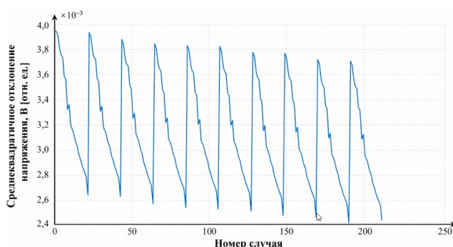
Рисунок 3. Отклонение напряжения по узлам для рассматриваемых сценариев
