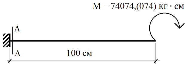
Рис. 5. К примеру 2. Расчетная схема
