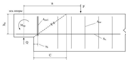
Рис. 1. Расчетная схема ригеля с подрезкой и положение наклонного сечения Т-1
