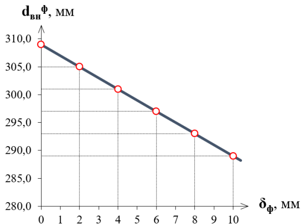
Рис. 2 График зависимости d_{вн}^{\phi}=f(\delta_{\phi})
