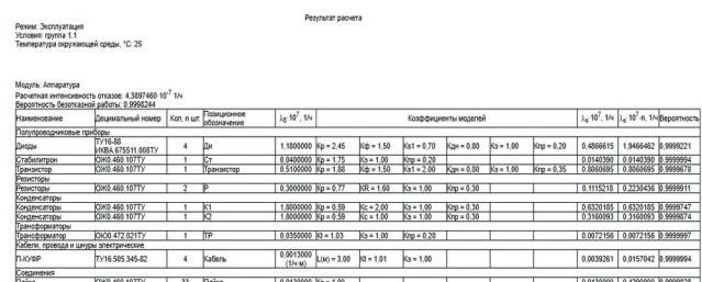
Рис. 11– Результат расчета регулируемого блока питания на стабилизтроне
